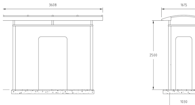
1304025 City 90 Traffic ladestasjon (1 modul) Ø90 stolpe, for 0 x 0 1 lader mm
