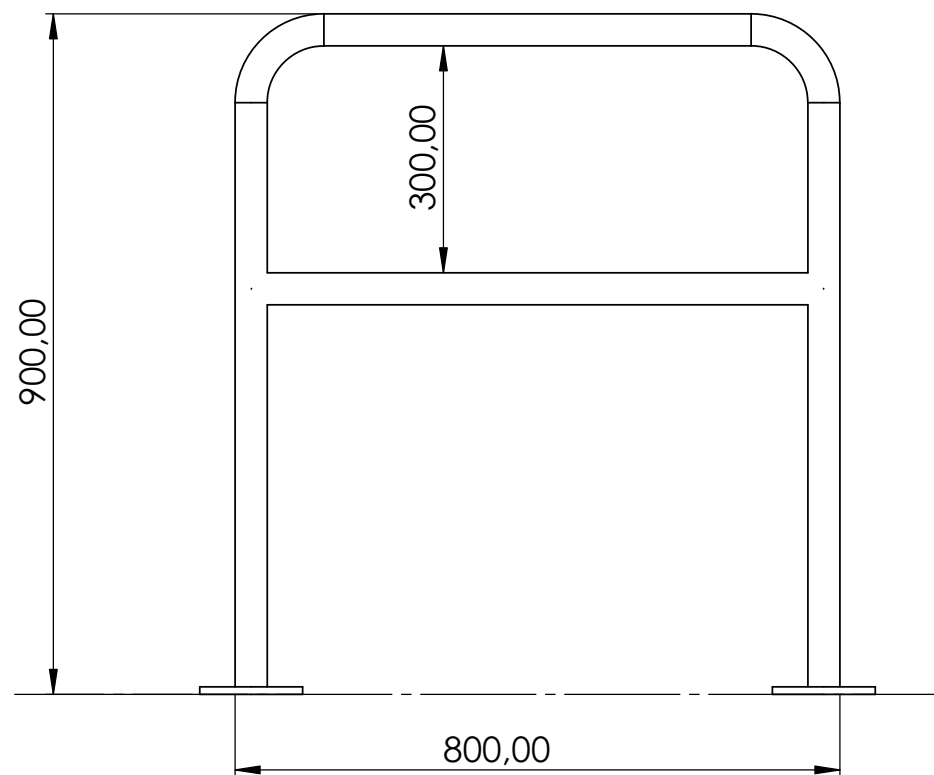
A-stativ for montering mot fundament Art: 1716 001
