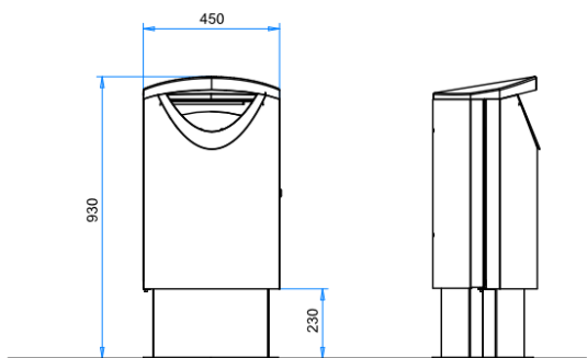
Ellipse 60L med forhøyet base.
