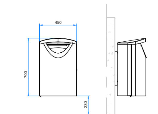
Ellipse 60L med innfestning for vegg.
