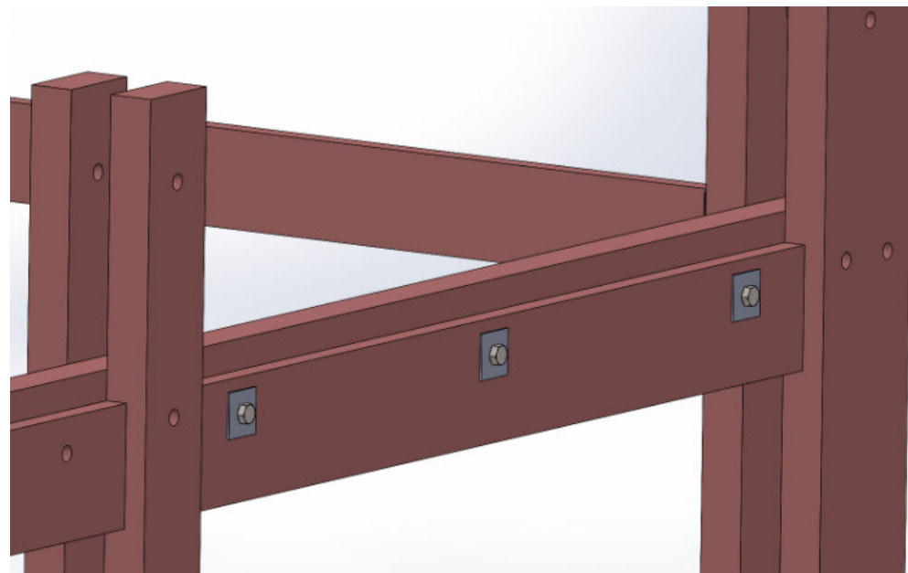
Hvordan forsterkningsplanke ser ut fra utsiden av leskuret.
