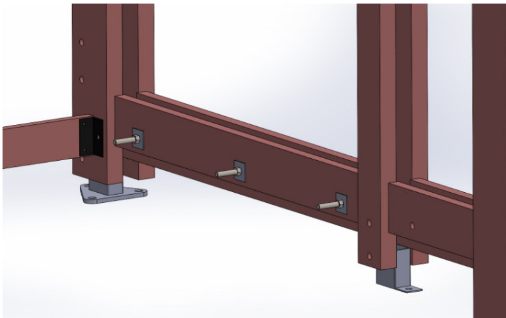
Hvordan forsterkningsplanke ser ut fra innsiden av leskuret
