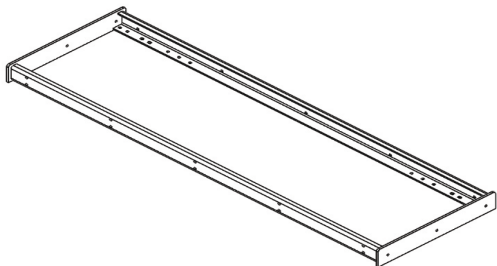
2 stk: ALG-003 Ben til benk
