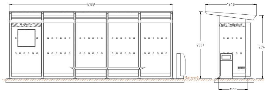
1801023 Moment med royalimpregnerert furu cc 1220 (5 felt) 6189 x 1940 mm
