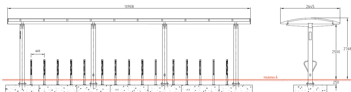
1305006 City 90 Piazza sykkelstall 3 modul 10908 x 2645 mm
