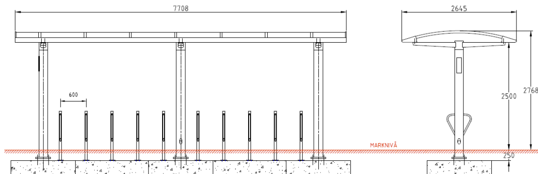
1305005 City 90 Piazza sykkelstall 2 modul 7708 x 2645 mm
