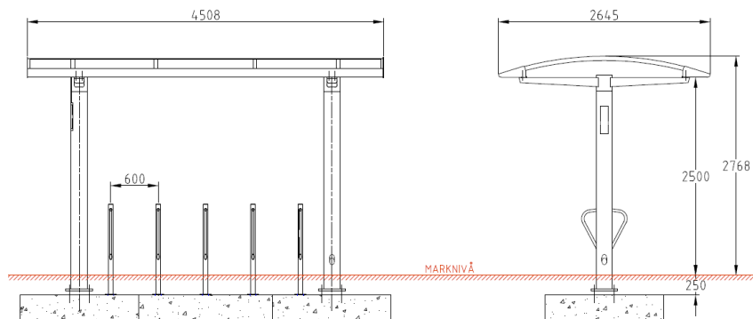
1305004 City 90 Piazza sykkelstall 1 modul 4508 x 2645 mm
