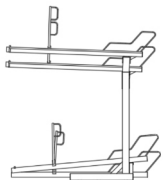
AX300-33L
