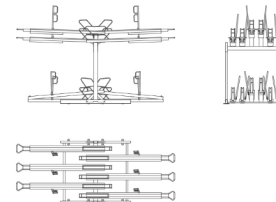
AX400-3333U
