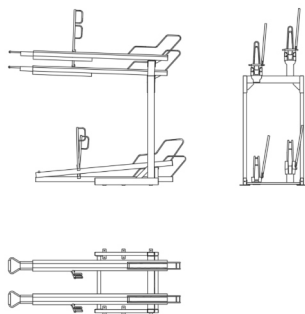
AX400-22UL
