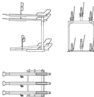
AX400-33UL
