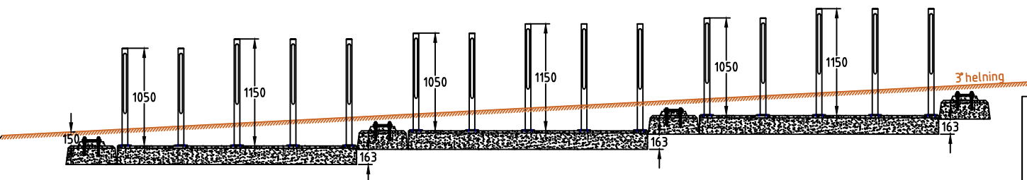
Eksempel på fundamentering ved hellende terreng, med tilpassede stolpelengder på sykkelstall og sykkelholdere.
