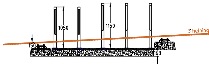
Eksempel på fundamentering ved hellende terreng, med tilpassede stolpelengder på sykkelstall og sykkelholdere.
